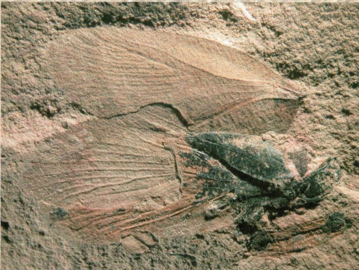
Блаттинопсида глафирифлебия и ее надкрылье
