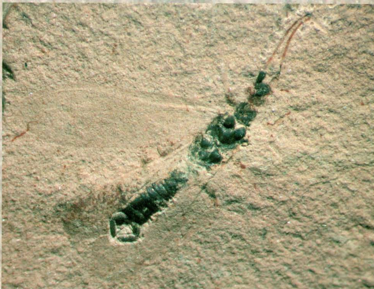
Цикадка и самец протоптеры трехмерной сохранности
