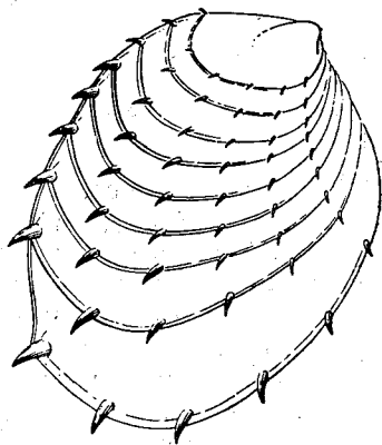
Рис. 118. Echinolimnadia mat- toxi Novojilov. L = 6,0 мм, па- ратип, реконструкция
