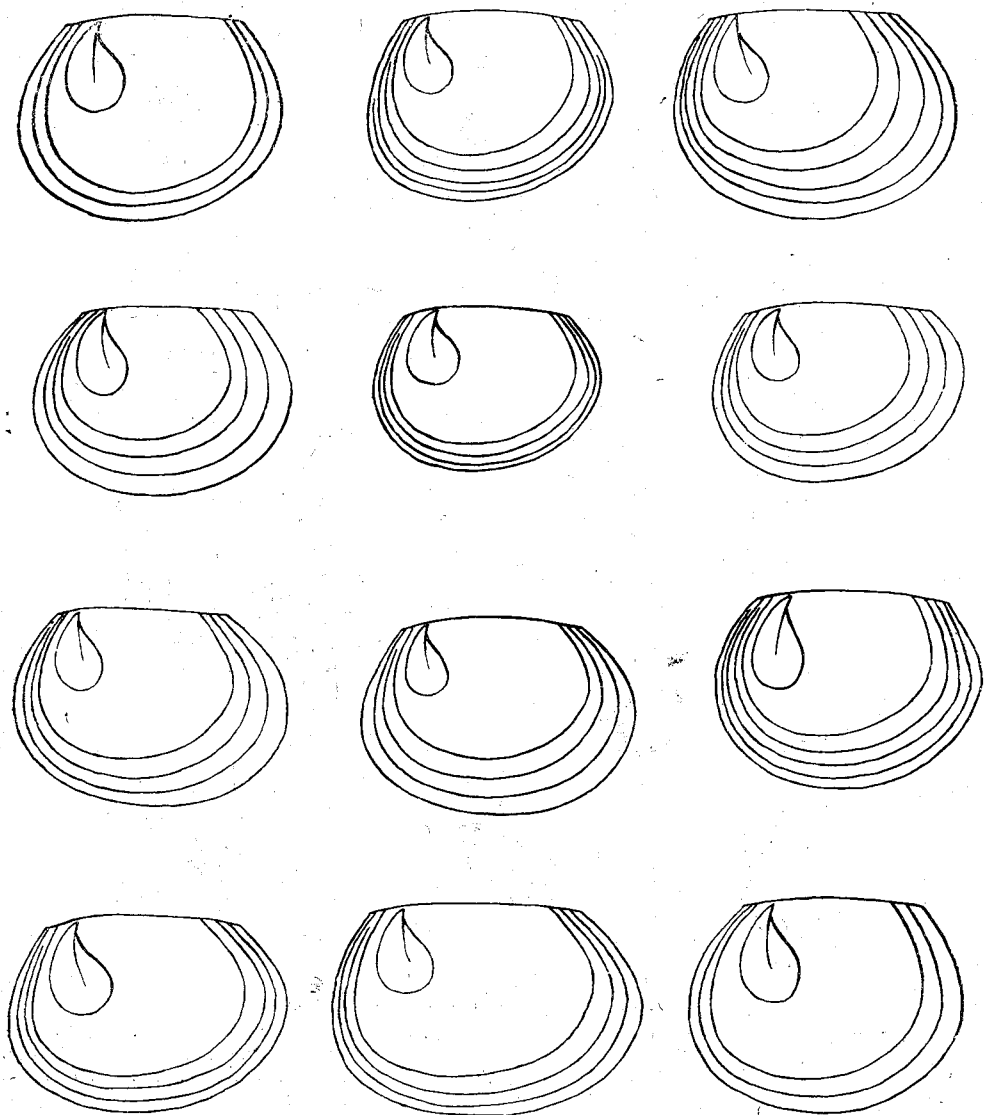
Рис. 4. Megasitum harmonicum Novojilov, gen. et sp. nov. Створки самцов и самок, показывающие постоянность формы и размещения бугра, очертания личиночных створок и створок раковины
