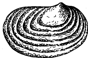
Рис. 120. Archaeosittum armoricanum (Novojilov). L = 3,8 мм
