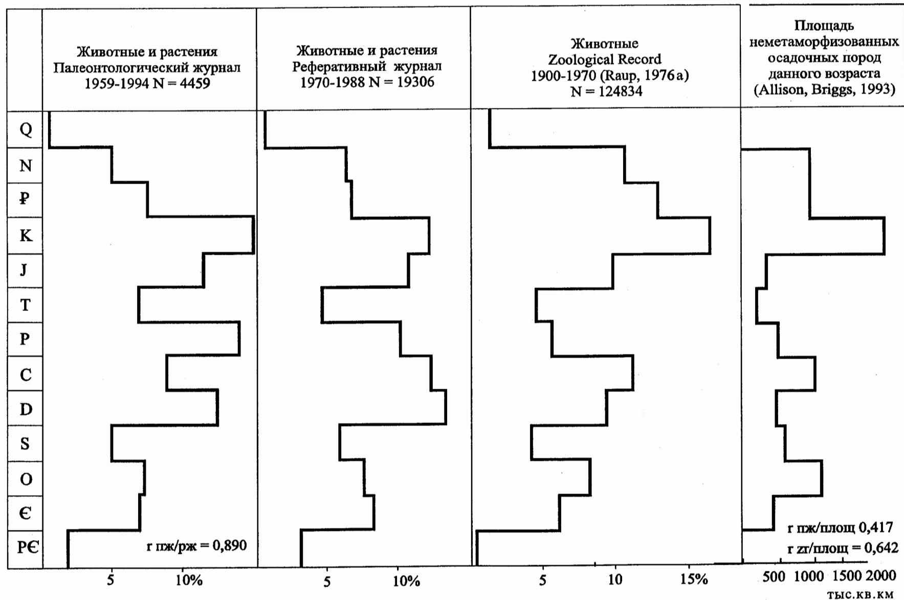
Рис. 3. Сравнение распределений по периодам числа новых видов животных и растений по данным различных источников и площади неметаморфизованных обнаженных осадочных пород
