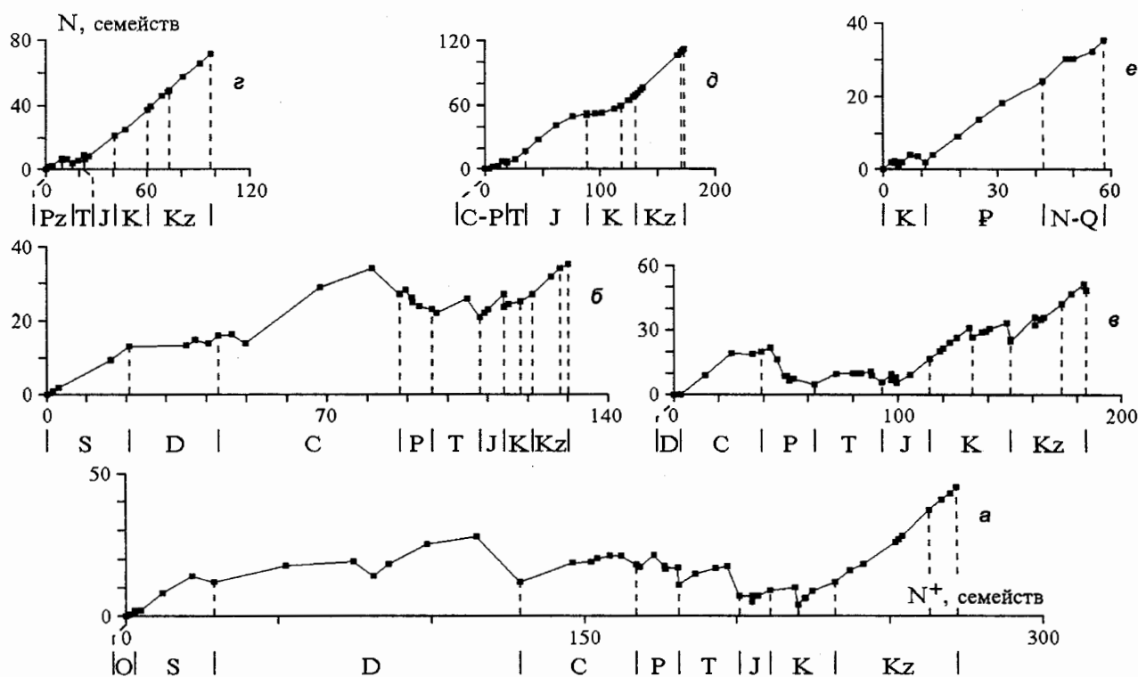
Рис. 29. Изменения разнообразия семейств основных крупных групп неморских водных животных в координатах число появившихся таксонов - мгновенное разнообразие: а - бесчелюстные и рыбы, б - членистоногие (кроме насекомых), в - тетраподы (кроме птиц), г - моллюски, д - насекомые, е - птицы
