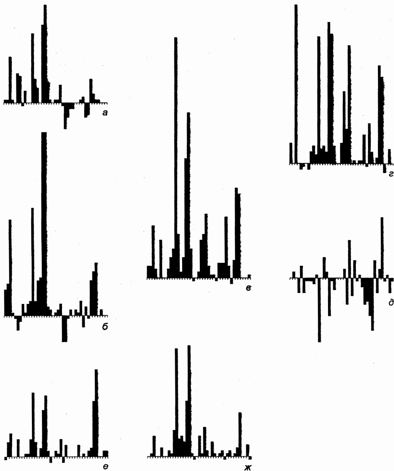
Рис. 22. Приращения числа родов в основных крупных группах морских животных в палеогене: а - даний, б - палеоцен, в - ипр, г - лютет, д - бартон и приабон, е - рюпель, ж - хатт. Основные группы слева направо: 1 - Spumellaria, 2 - Nassellaria, 3 - Foraminifera, 4 - прочие Protozoa, 5 - Porifera, 6 - Scleractinia, 7 - прочие Coelenterata, 8 - Annelida, 9 - Nuculoida, 10 - Arcoida, 11 - Pterioida, 12 - Veneroida, 13 - прочие Bivalvia, 14 - Archaeogastropoda, 15 - Heterostrophia, 16 - Mesogastropoda, 17 - Neogastropoda, 18 - прочие Gastropoda, 19 - Cephalopoda, 20 - прочие Mollusca, 21 - Cirripedia, 22 - Malacostraca, 23 - Ostracoda, 24 - Cheilostomata, 25 - прочие Bryozoa, 26 - Terebratulida, 27 - прочие Brachiopoda, 28 - «Pelmatozoa», 29 - Temnopleuroidea, 30 - Clypeasteroidea, 31 - Cassiduloida, 32 - Spatangoida, 33 - прочие Echinoidea, 34 - прочие «Eleutherozoa», 35 - Chondrichthyes, 36 - Perciformes, 37 - прочие Osteichthyes, 38 - Reptilia, 39 - Aves, 40 - Cetacea, 41 - прочие Mammalia
