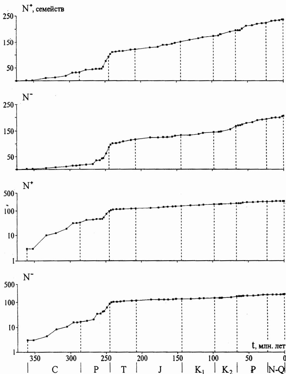
Рис. 44. Появление (а, в) и вымирание (б, г) семейств неморских водных и амфибиотических тетрапод: а, б - в обычных координатах, в, г - в полулогарифмических координатах
