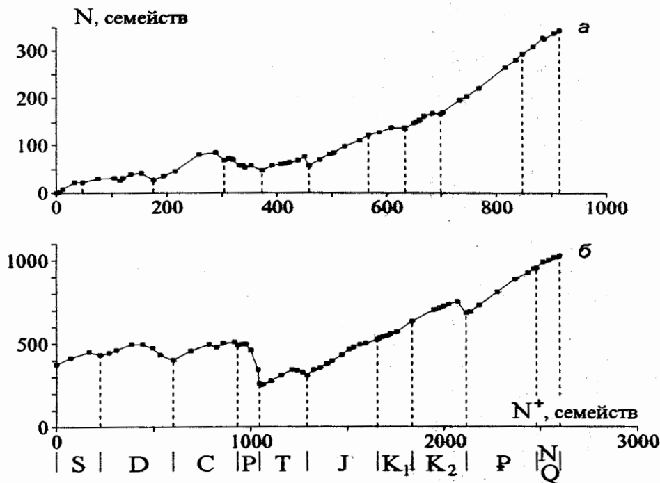
Рис. 26. Изменения разнообразия животных в морской и континентальной водной биоте в координатах число появившихся семейств - мгновенное число семейств: а - неморская биота; б - морская биота.
