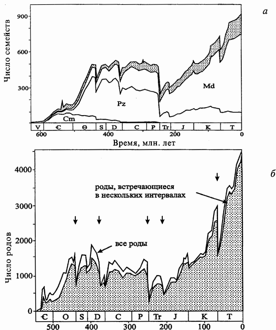
Рис. 45. Эволюция разнообразия морских животных в фанерозое: а - изменения глобального числа семейств с выделением кембрийской, палеозойской и современной великих эволюционных фаун (Sepkoski, 1982), б - изменения глобального числа родов (Sepkoski, 1996). Временная шкала по Harland et al. , 1990
