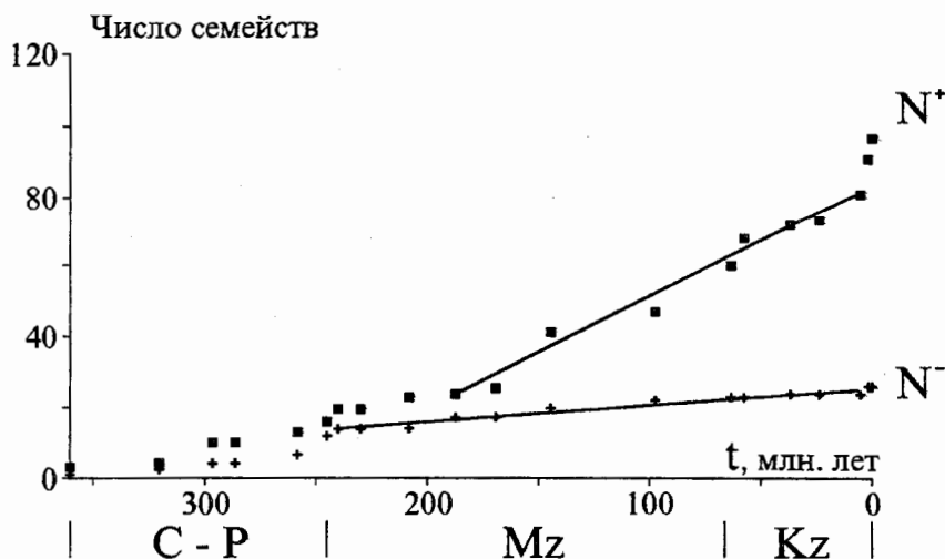
Рис. 30. Появление и вымирание семейств пресноводных моллюсков; N^+ - число появившихся семейств, N^- - число вымерших семейств
