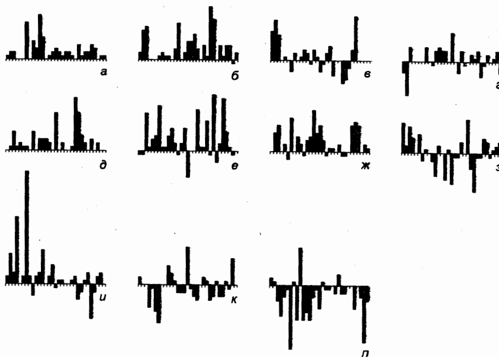
Рис. 20. Приращения числа родов в основных крупных группах морских животных в юре; а - геттанг, б - синемюр, в - плинсбах, г - тоар, д - аален, е - байос, ж - бат, з - келловей, и - оксфорд, к - кимеридж, л - титон. Основные группы слева направо: 1 - Spumellaria, 2 - Nassellaria, 3 - Foraminifera, 4 - Demospongia, 5 - Calcarea, 6 - Hexactinellida, 7 - Coelenterata, 8 - Annelida, 9 - Pterioidea, 10 - Trigonioidea, 11 - Veneroidea, 12 - прочие Bivalvia, 13 - Archaeogastropoda, 14 - Mesogastropoda, 15 - прочие Gastropoda, 16 - Ammonoidea, 17 - прочие «Ectocochlia», 18 - Coleoidea, 19 - Podocopida, 20 - прочие Ostracoda, 21 - прочие Arthropoda, 22 - Bryozoa, 23 - Rhynchonellida, 24 - Terebratulida, 25 - прочие Brachiopoda, 26 - «Pelmatozoa», 27 - Echinoidea, 28 - прочие «Eleutherozoa», 29 - Chondrichthyes, 30 - Osteichthyes, 31 - Reptilia
