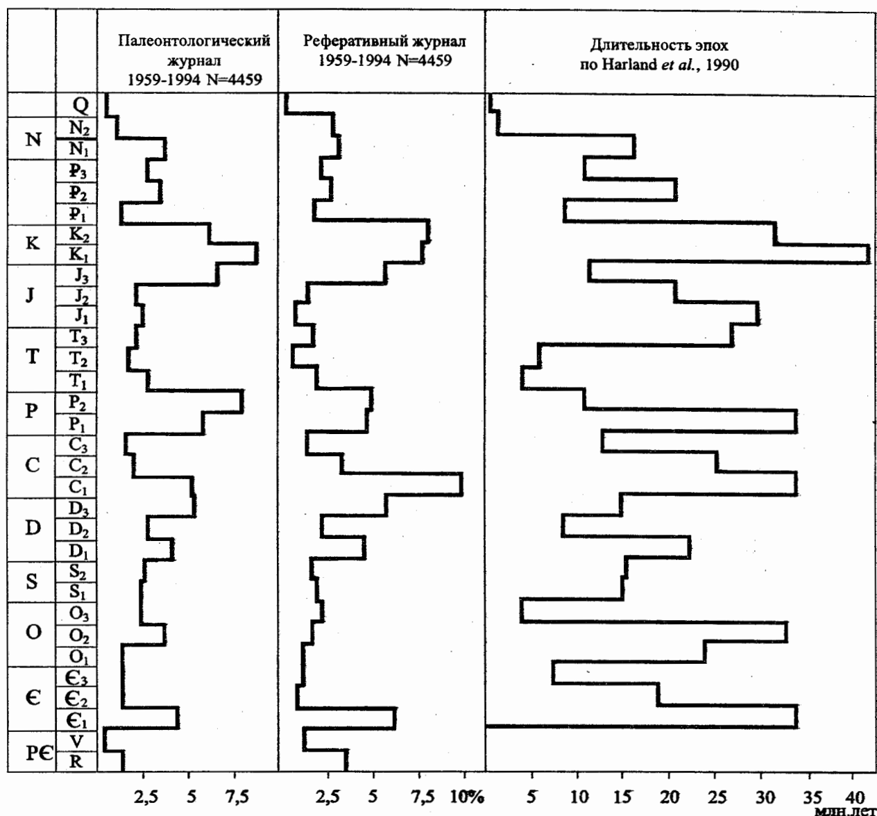
Рис. 4. Сравнение распределений по эпохам числа новых видов животных и растений по данным различных источников и длительности эпох по шкале Harland et al. , 1990
