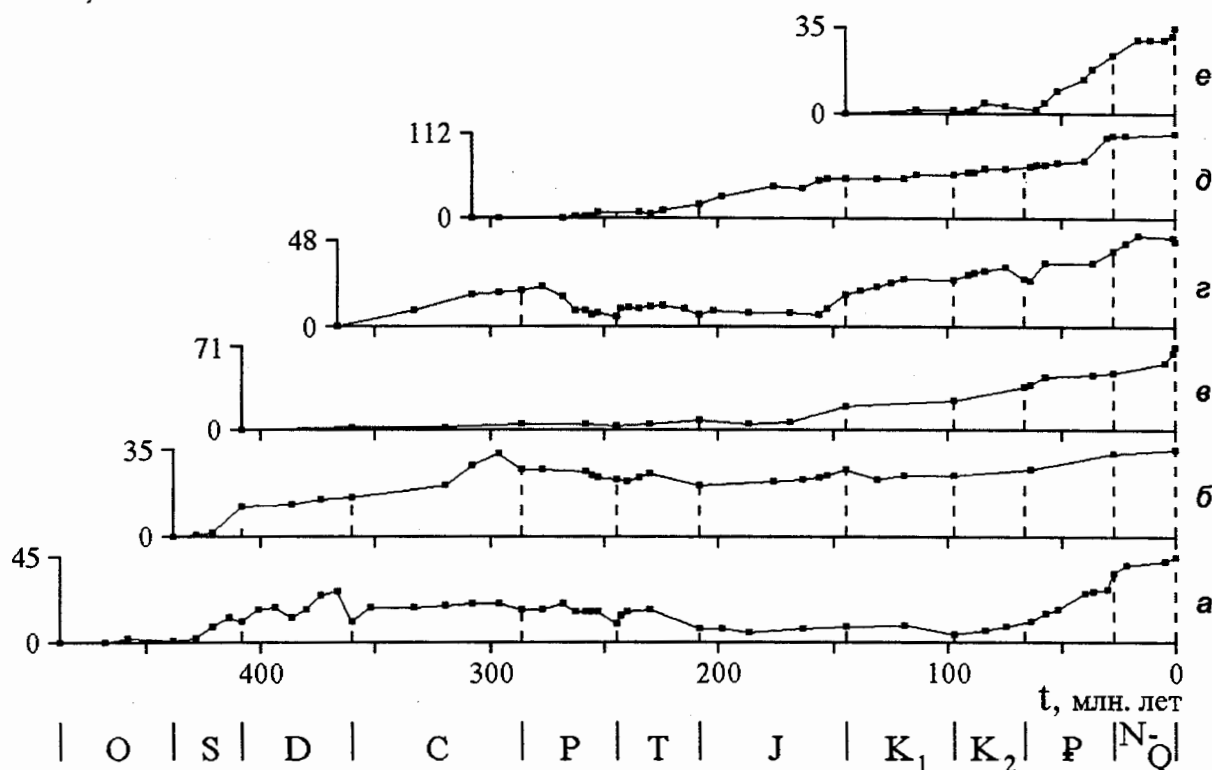
Рис. 28. Изменения разнообразия семейств основных крупных групп неморских водных животных в координатах время - мгновенное разнообразие (Дмитриев и др., 1995): а - асцелулятные и рыбы, б - членистоногие (кроме насекомых), в - моллюски, г - тетраподы (кроме птиц), д - насекомые, е - птицы
