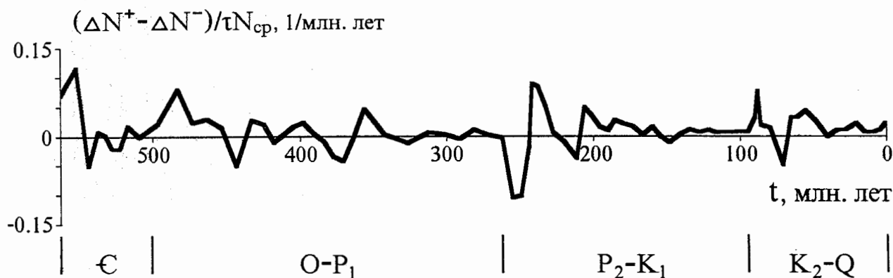
Рис. 12. Удельная скорость изменения числа родов морских животных в фанерозе
