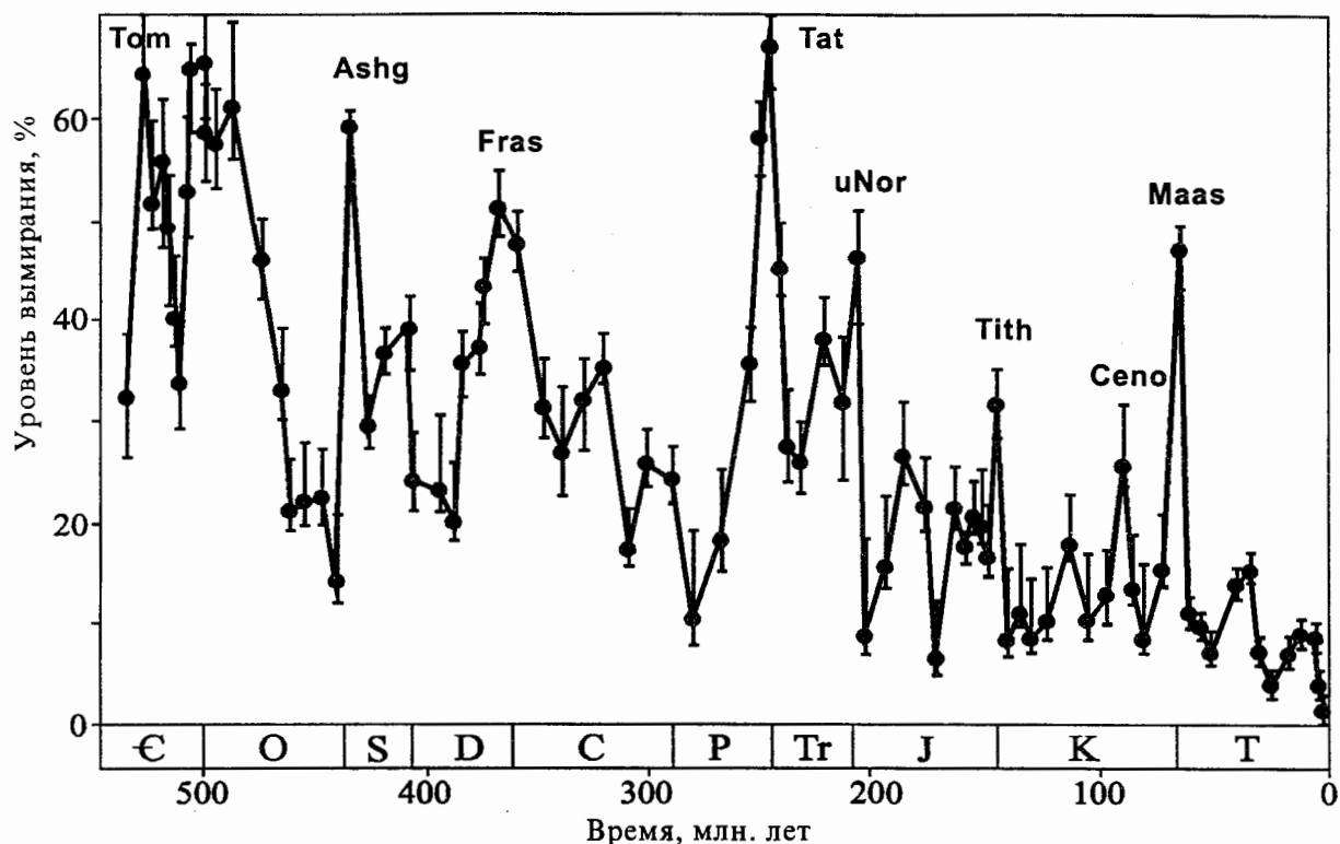
Рис. 48. Изменения уровня вымирания родов морских животных на протяжении кембрия - неогена (Sepkoski, 1996). Массовые вымирания: Tom - томмотское, Ashg - ашгиллское, Fras - франское, Tat - позднепермское, uNor - поздненорийское, Tith - титонское, Ceno - сеноманское, Maas - маастрихтское. Временная шкала по Harland et al. , 1990
