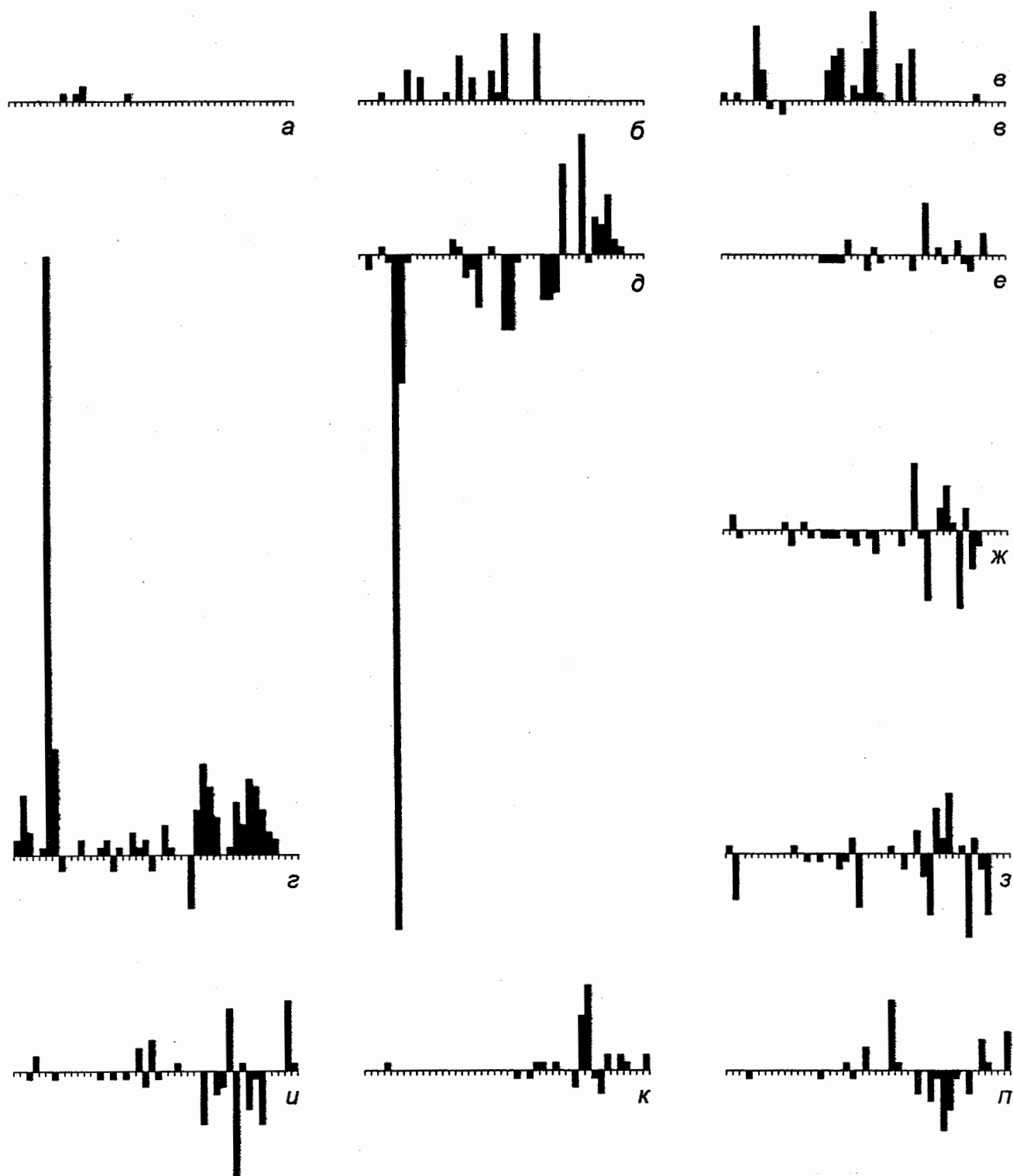
Рис. 15. Приращения числа родов в основных крупных группах морских животных в позднем венде и кембрии; а - поздний венд, б - немакит-далдын, в - томмот, г - атдабан, д - конец раннего кембрия, е-з - средний кембрий: е - начало, ж - середина, з - конец, и - дресбач, к - франкон, л - тремпельон. Основные группы слева направо: 1 - Protozoa, 2 - Demospongia, 3 - Calcareia, 4 - Hexactinellida, 5 - Porifera inc. cl., 6 - Regulares, 7 - Irregulares, 8 - Trilobozoa, 9 - Cyclozoa, 10 - Scyphozoa, 11 - Hydrozoa, 12 - Anthozoa, 13 - Coelenterata inc. sed., 14 - Chaetognatha, 15 - Annelida, 16 - Coeloscleritophora, 17 - Tommotiida, 18 - Machaeridia, 19 - прочие Problematica, 20 - Tergomya, 21 - Helcionelloida, 22 - Rostroconchia, 23 - Orthothecimorpha, 24 - Hyolithomorpha, 25 - Bivalvia, 26 - Gastropoda, 27 - Cephalopoda, 28 - прочие Mollusca, 29 - Olenellida, 30 - Agnostida, 31 - Redlichiida, 32 - Corynexochida, 33 - Odontopleurida, 34 - Asaphida, 35 - Ptychopariida, 36 - прочие Trilobita, 37 - Ostracoda, 38 - прочие Arthropoda, 39 - Inarticulata, 40 - Articulata, 41 - Echinodermata, 42 - Pterobranchia, 43 - Graptolithina, 44 - Conodonta
