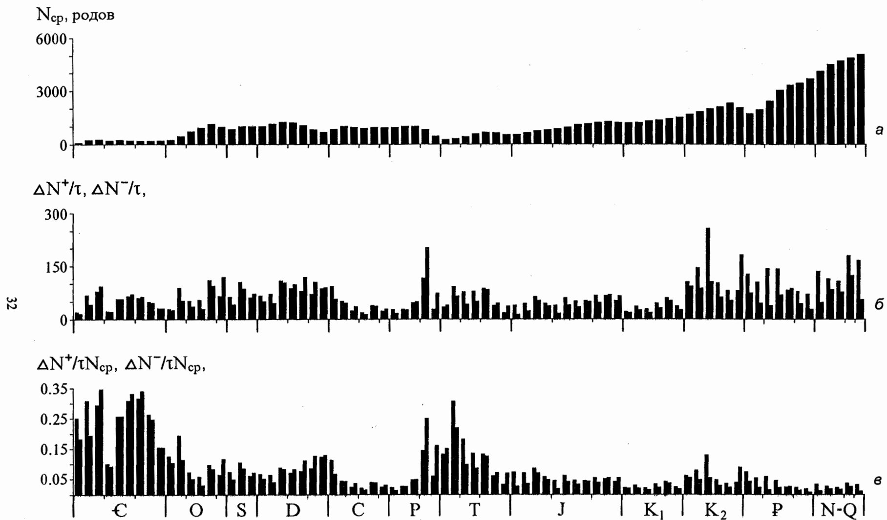
Рис. 11. Среднее мгновенное разнообразие и скорости появления и вымирания родов морских животных по векам фанерозоя: а - среднее мгновенное разнообразие (метрика Вебба-Харпера), б - скорости, в - удельные скорости. На диаграммах скоростей даны пары столбцов по векам, левый столбец относится к появлению родов, правый - к вымиранию
