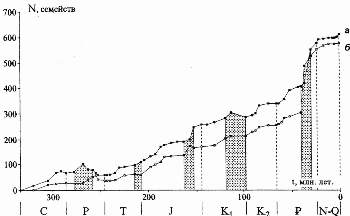
Рис. 13. Сопоставление кривых числа семейств ископаемых насекомых: а - по данным Labandeira, 1994, б - данные Лаборатории членистоногих ПИН. Тениями выделены интервалы наиболее существенных несовпадений. Объяснения в тексте
