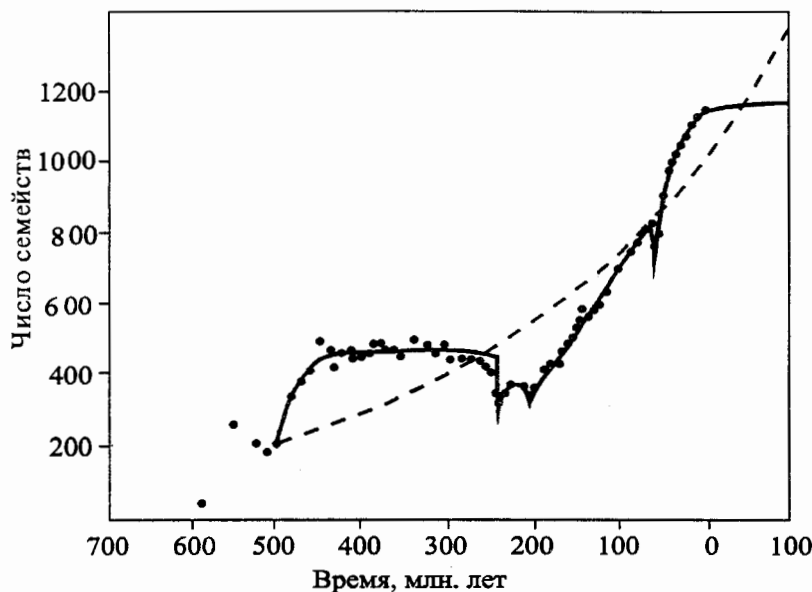
Рис. 46. Изменения числа семейств морских организмов в венде и фанерозе. Пунктирной линией показана экспоненциальная аппроксимация зависимости между уровнем семейственного разнообразия и геологическим временем, сплошной линией — поsegmentная логистическая аппроксимация. По Courtillot, Gaudemer, 1996, с изменениями
