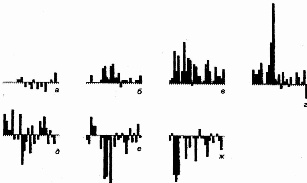
Рис. 19. Приращения числа родов в основных крупных группах морских животных в триасе; а - инд, б - оленек, в - анизий, г - ладин, д - карний, е - норий, ж - рэт. Основные группы слева направо: 1 - Spumellaria, 2 - Nassellaria, 3 - Foraminifera, 4 - Porifera, 5 - Scleractinia, 6 - прочие Coelenterata, 7 - Polychaeta, 8 - Pterioidea, 9 - прочие Bivalvia, 10 - Archaeogastropoda, 11 - Mesogastropoda, 12 - прочие Gastropoda, 13 - Nautilida, 14 - Ceratitida, 15 - прочие Cephalopoda, 16 - Ostracoda, 17 - прочие Arthropoda, 18 - Bryozoa, 19 - Rhynchonellida, 20 - Spiriferida, 21 - Terebratulida, 22 - прочие Brachiopoda, 23 - Crinoidea, 24 - Holothuroidea, 25 - прочие «Eleutherozoa», 26 - Conodonta, 27 - Chondrichthyes, 28 - Reptilia
