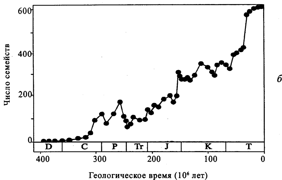
Рис. 31. Число семейств насекомых, существование которых выявлено в течение: а - эпох (Jarzembowski, Ross, 1993), б - веков (Labandeira, Sepkoski, 1993)
